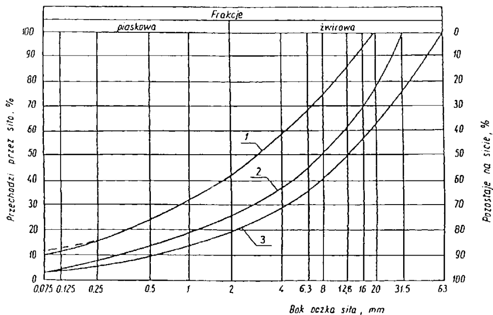
Rysunek 1. Pole na podbudowy dobrego uziarnienia kruszyw przeznaczonych wykonywane metodą stabilizacji mechanicznej
